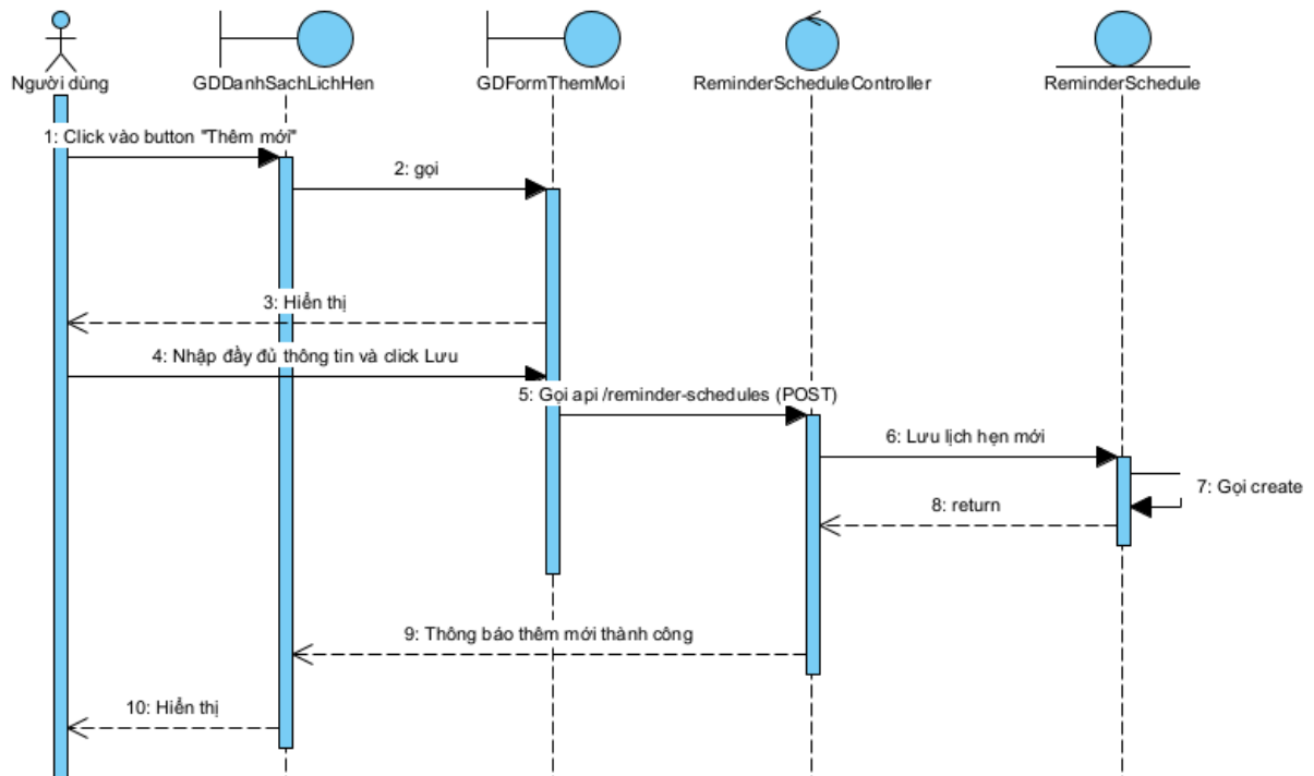
Hình 2.43 Biểu đồ tuần tự chức năng thêm lịch hẹn
