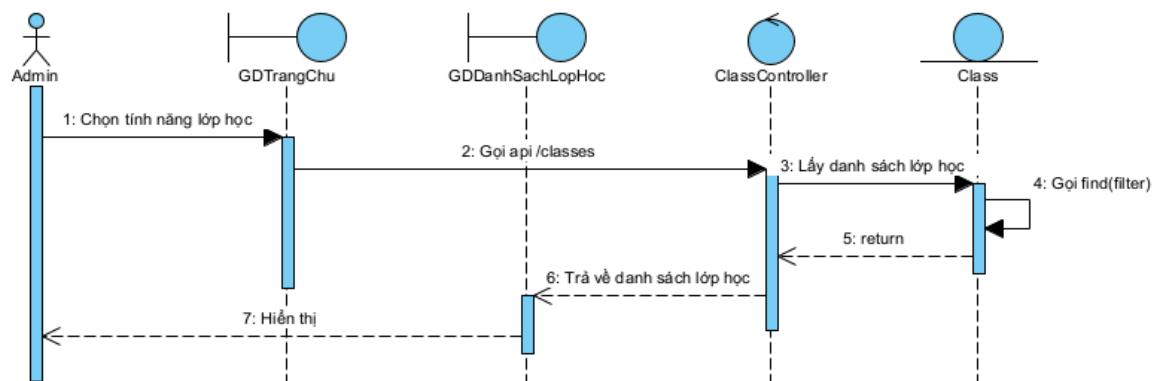
Hình 2.65 Biểu đồ tuần tự chức năng xem danh sách lớp học
