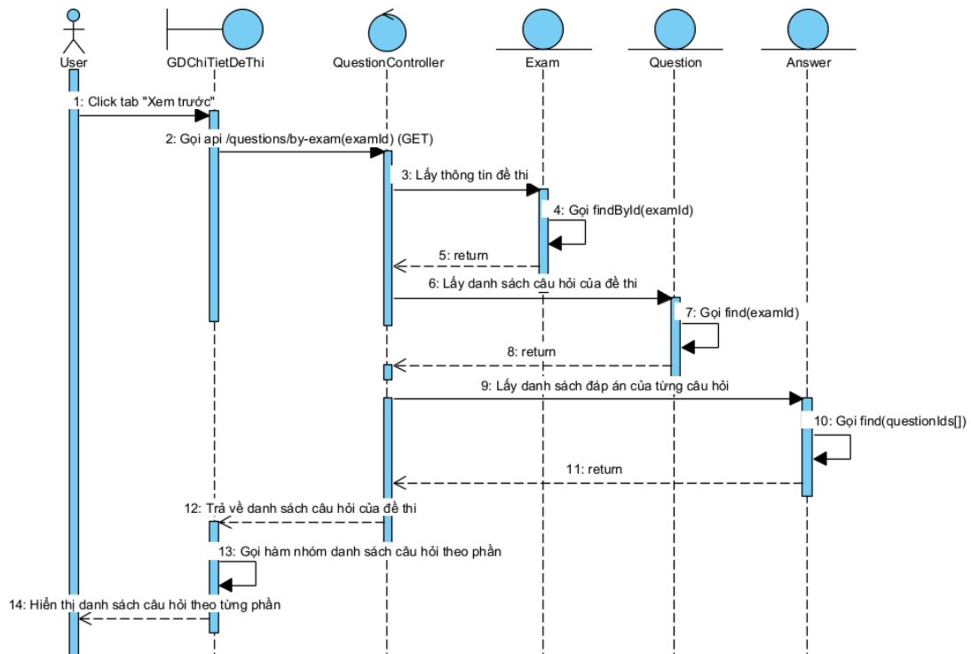
Hình 2.34 Biểu đồ tuần tự chức năng xem trước đề thi trên App
