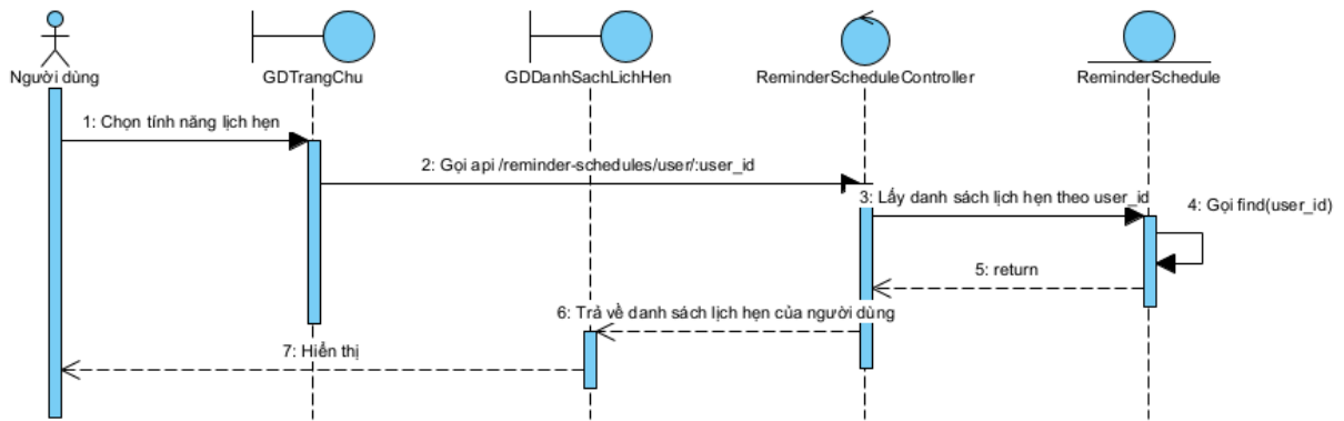
Hình 2.42 Biểu đồ tuần tự chức năng xem danh sách lịch hẹn
