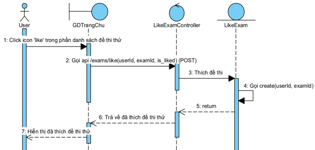
Hình 2.29 Biểu đồ tuần tự chức năng thích đề thi thử
