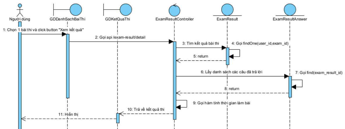
Hình 2.39 Biểu đồ tuần tự chức năng xem kết quả thi
