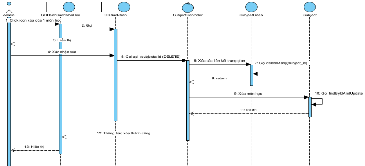
Hình 2.64 Biểu đồ tuần tự chức năng xóa môn học
