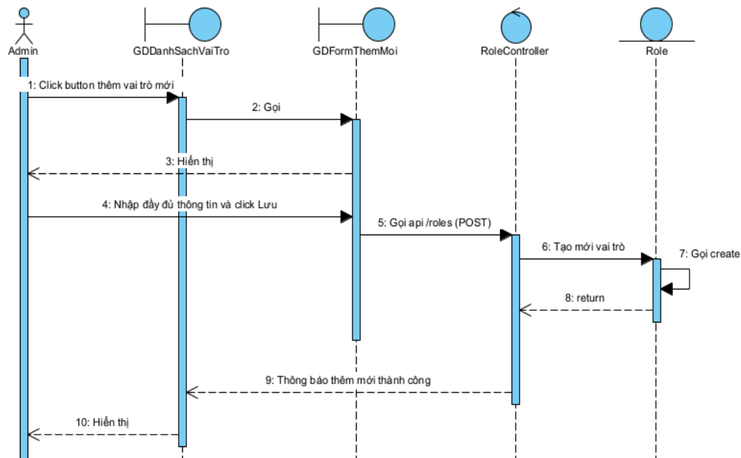
Hình 2.52 Biểu đồ tuần tự chức năng thêm vai trò
