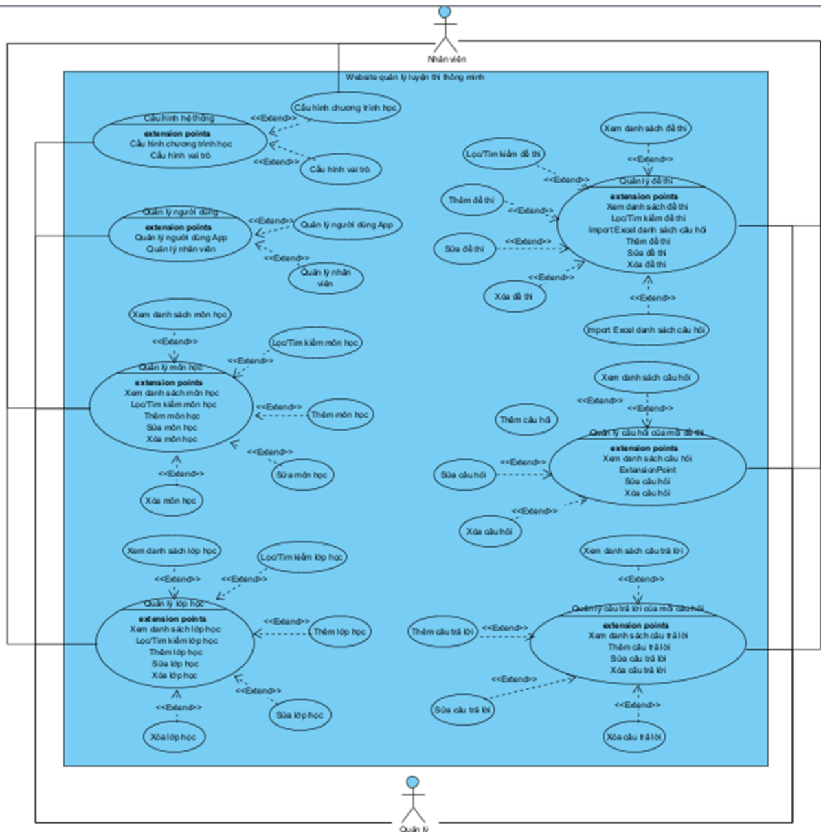
Hình 2.2 Biểu đồ use case tổng quát của website quản lý luyện thi
