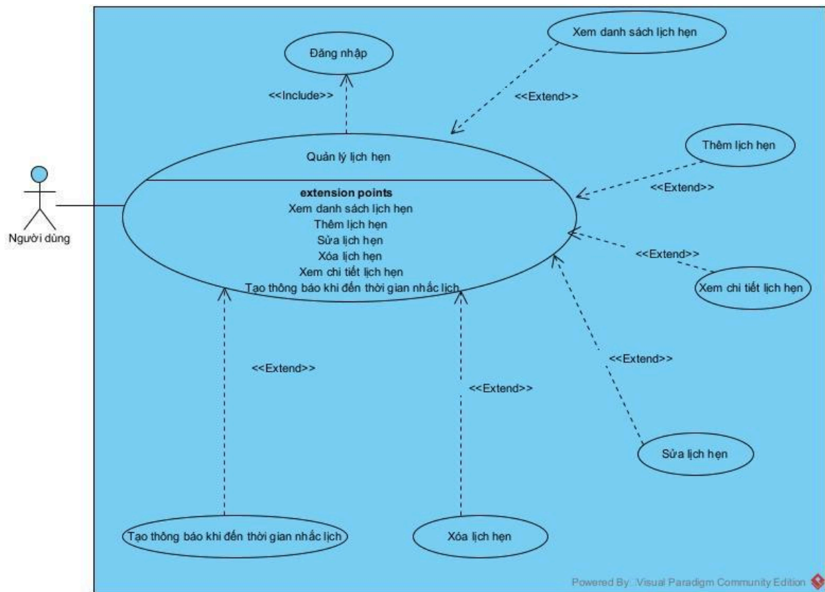
Hình 2.13 Biểu đồ use case chi tiết module quản lý lịch hẹn
