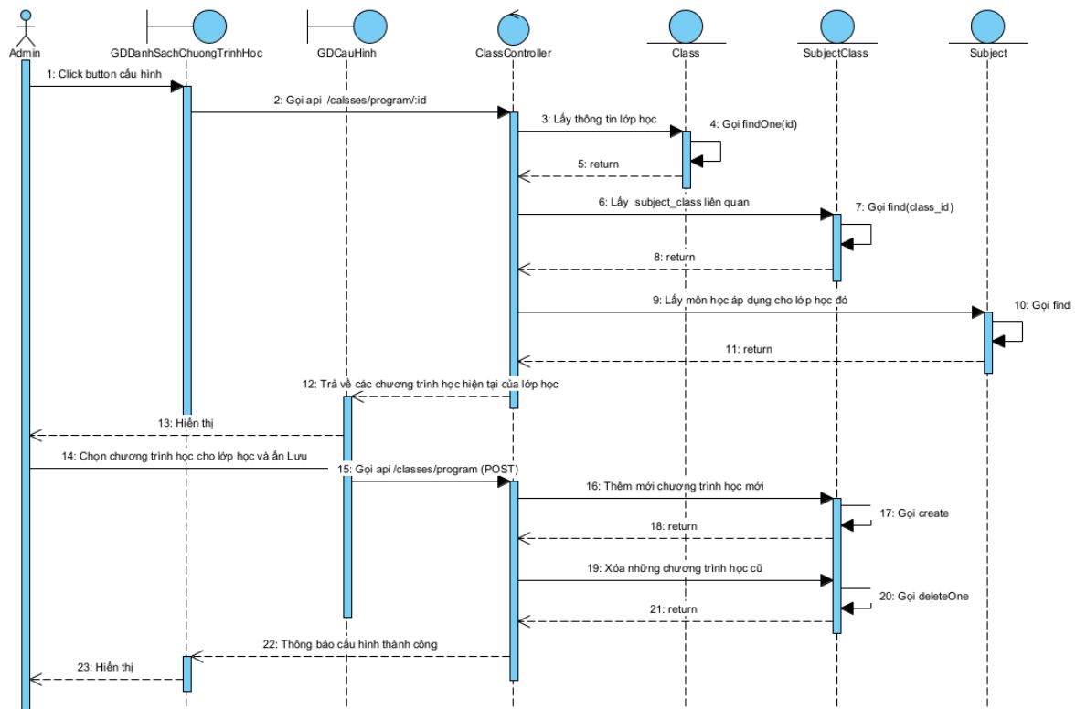
Hình 2.57 Biểu đồ tuần tự chức năng cấu hình chương trình học
