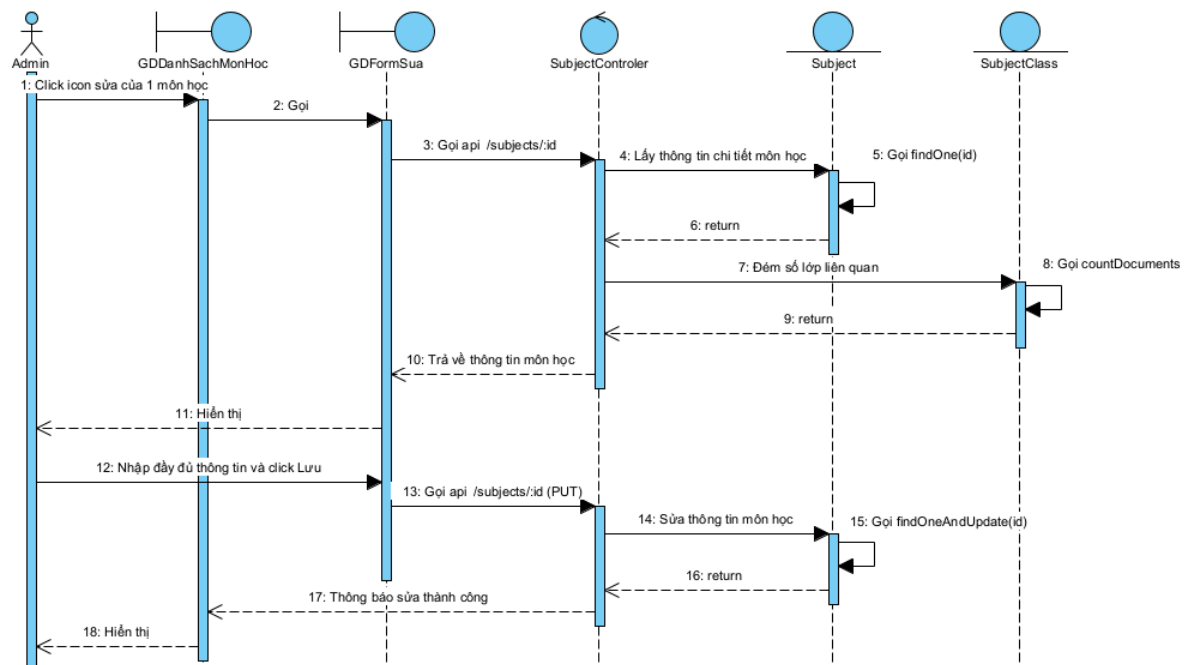
Hình 2.63 Biểu đồ tuần tự chức năng sửa môn học
