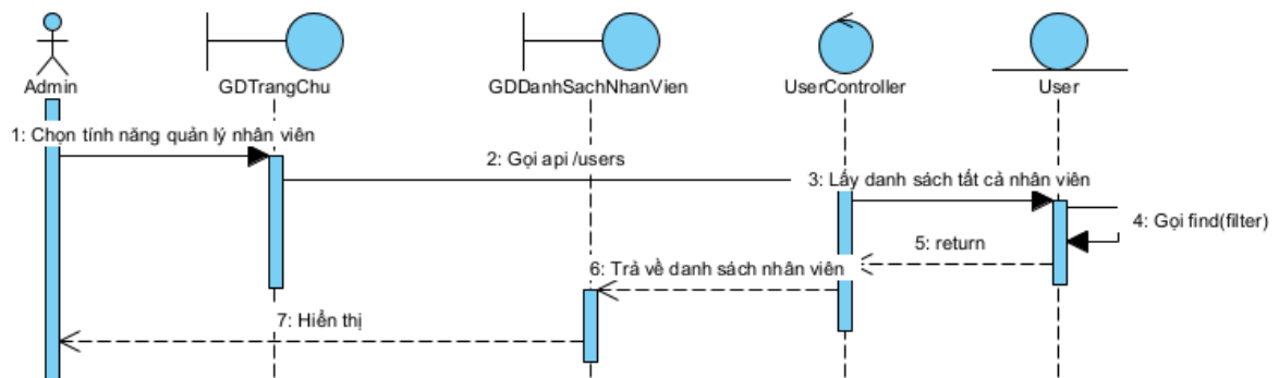
Hình 2.58 Biểu đồ tuần tự chức năng xem danh sách nhân viên
