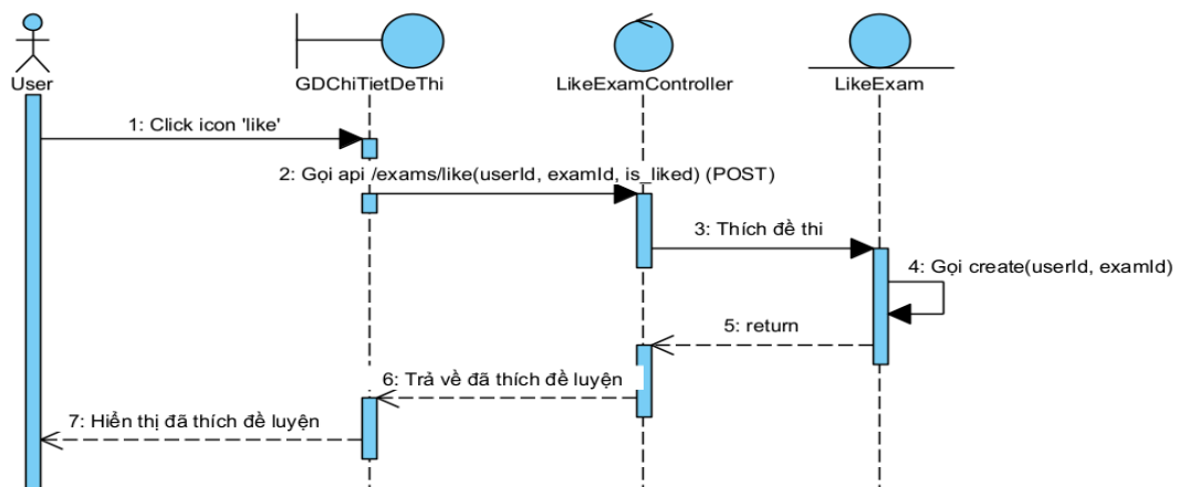
Hình 2.29 Biểu đồ tuần tự chức năng thích đề thi thử
