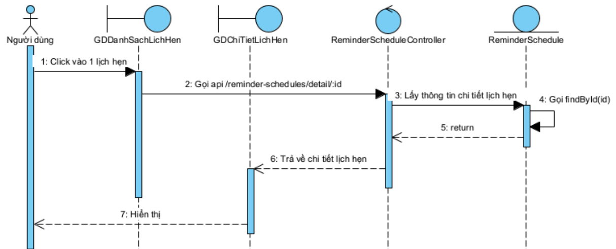
Hình 2.44 Biểu đồ tuần tự chức năng xem chi tiết lịch hẹn
