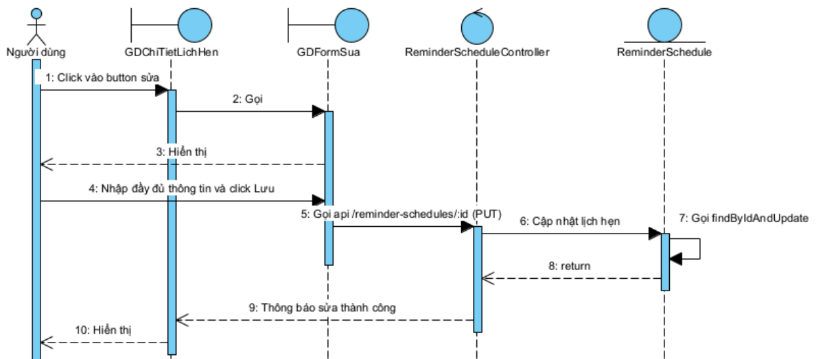
Hình 2.45 Biểu đồ tuần tự chức năng sửa lịch hẹn
