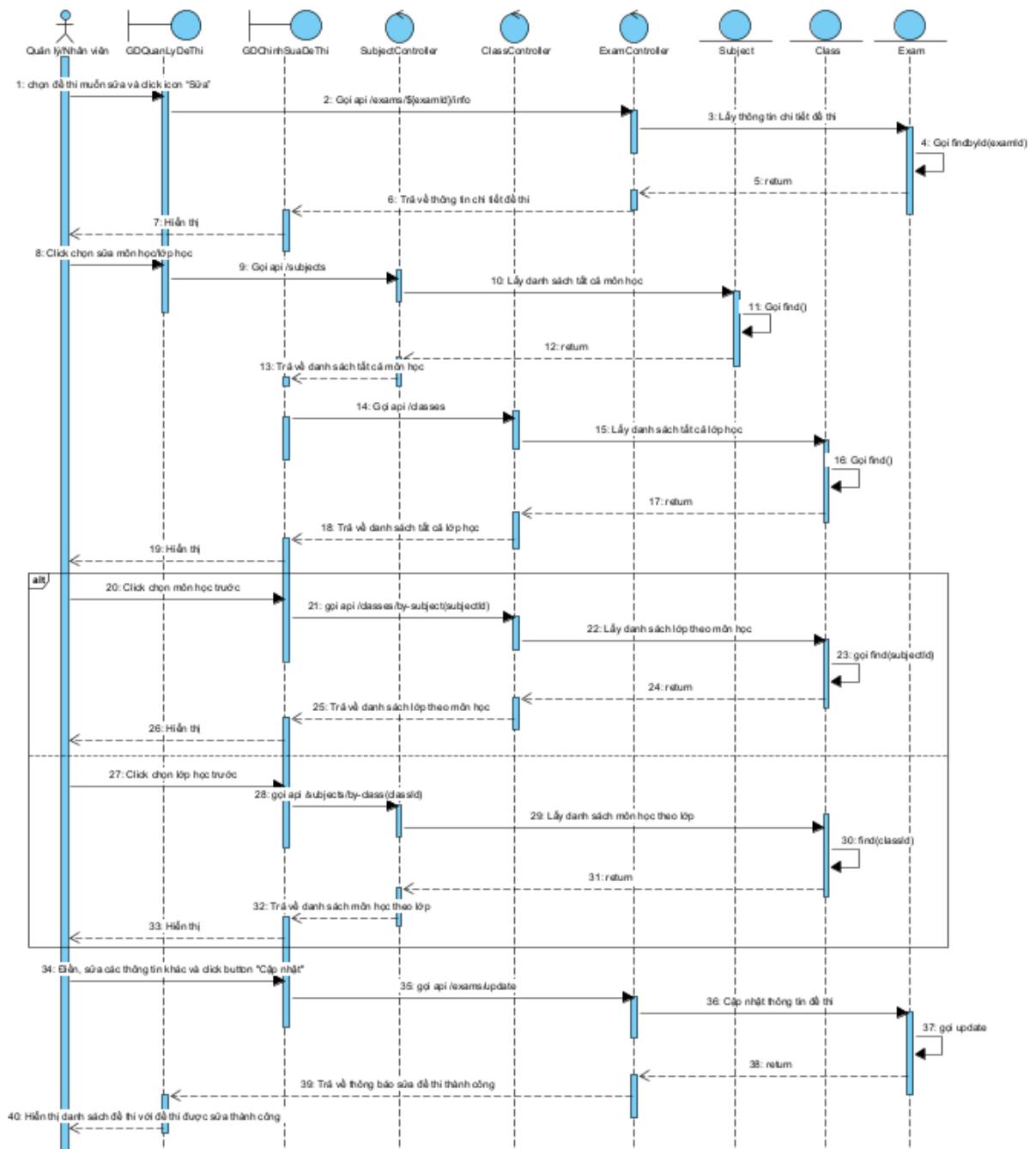
Hình 2.71 Biểu đồ tuần tự chức năng sửa đề thi
