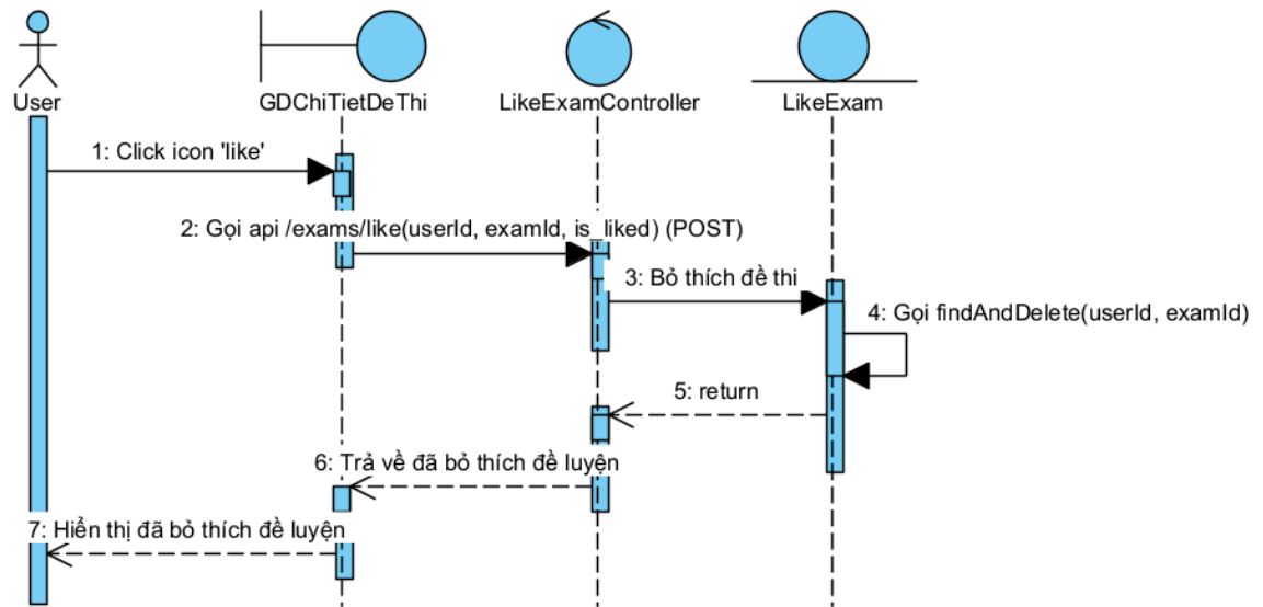
Hình 2.32 Biểu đồ tuần tự chức năng bỏ thích đề luyện
