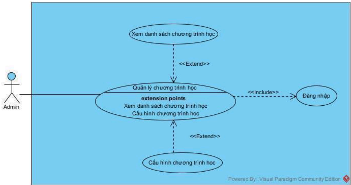
Hình 2.16 Biểu đồ use case chi tiết module quản lý chương trình học
