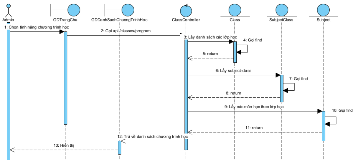
Hình 2.56 Biểu đồ tuần tự chức năng xem danh sách chương trình học
