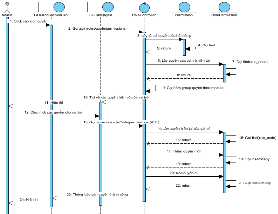
Hình 2.55 Biểu đồ tuần tự chức năng gán quyền cho vai trò
