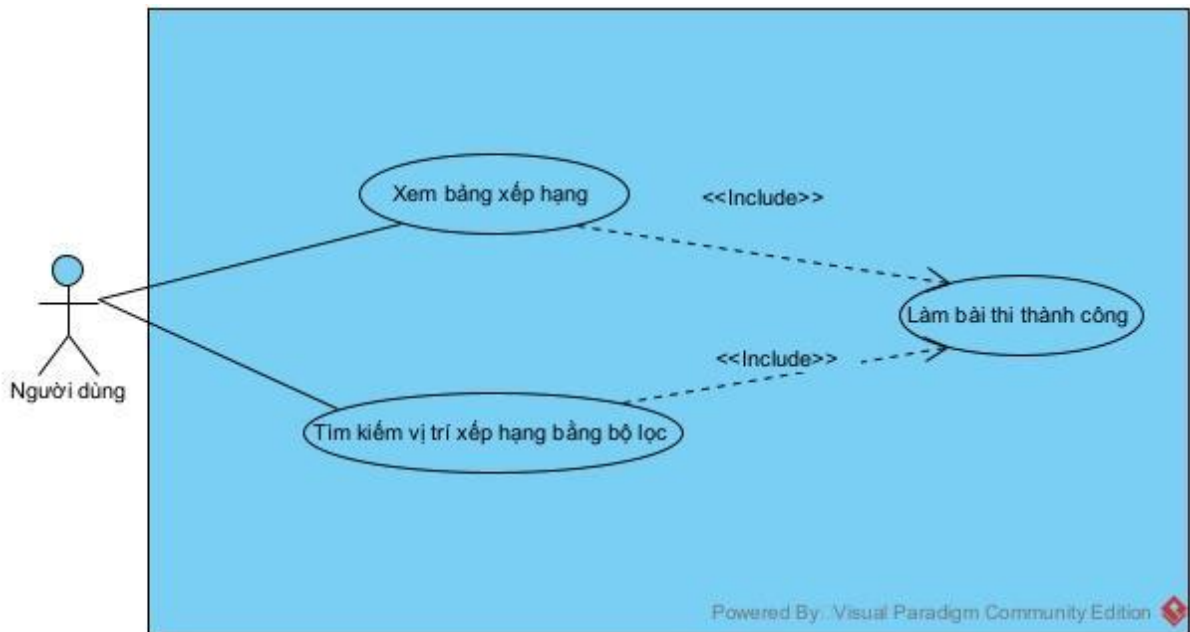
Hình 2.12 Biểu đồ use case chi tiết module xem bảng xếp hạng của bài thi thử
