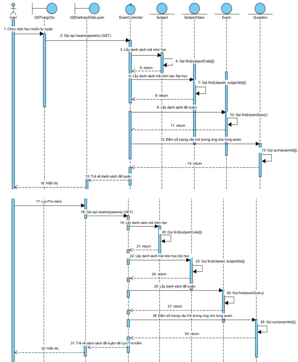
Hình 2.25 Biểu đồ tuần tự chức năng xem danh sách đề luyện
