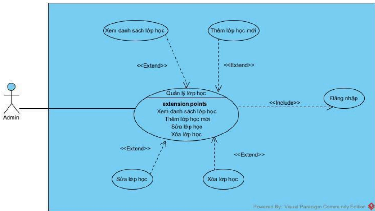
Hình 2.19 Biểu đồ use case chi tiết module quản lý lớp học
