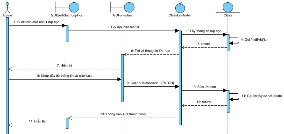
Hình 2.67 Biểu đồ tuần tự chức năng sửa lớp học
