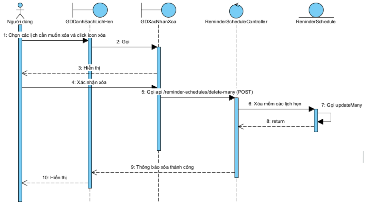
Hình 2.46 Biểu đồ tuần tự chức năng xóa lịch hẹn
