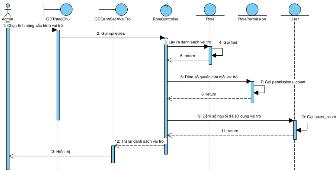
Hình 2.51 Biểu đồ tuần tự chức năng xem danh sách vai trò
