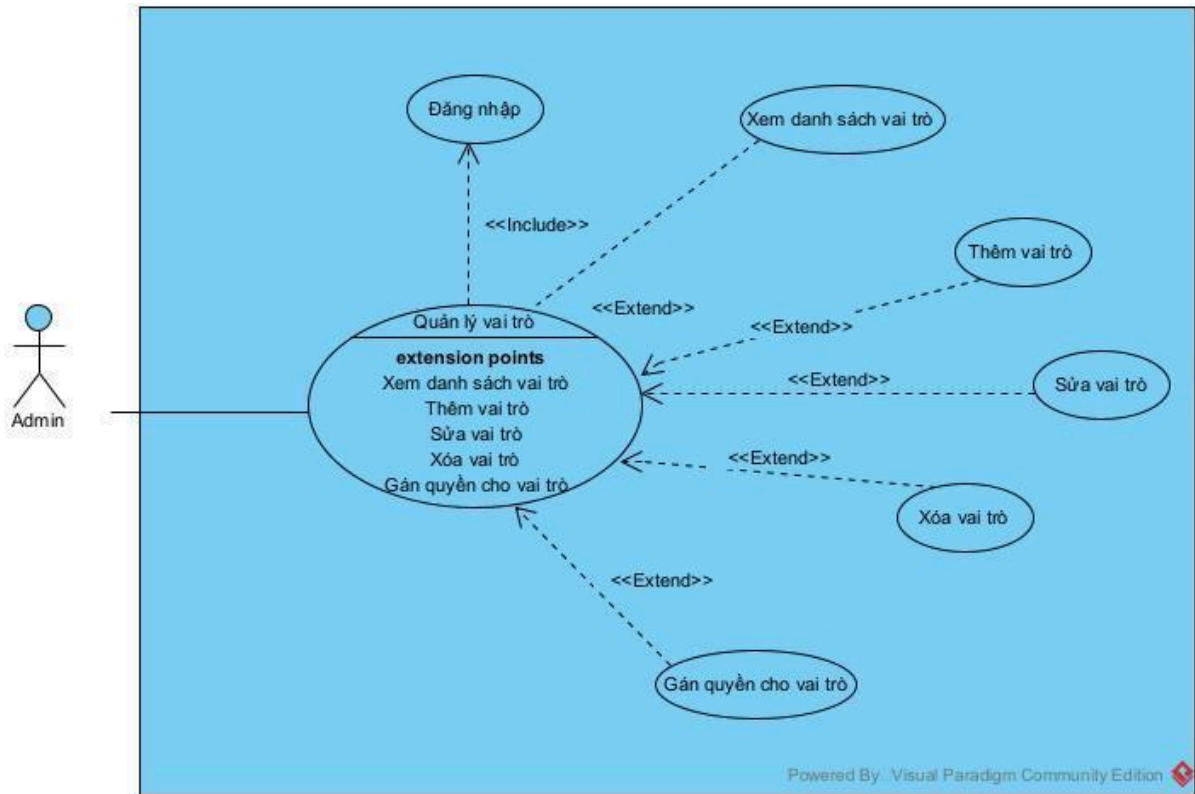
Hình 2.15 Biểu đồ use case chi tiết module quản lý vai trò
