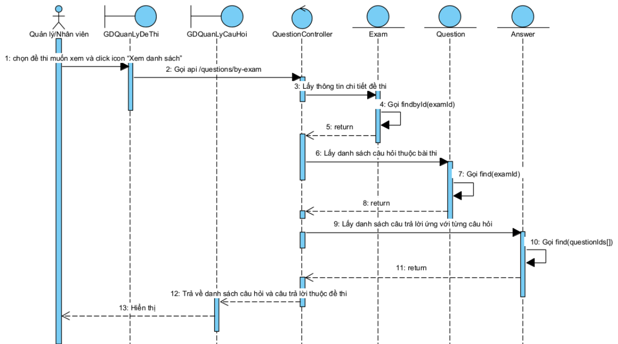
Hình 2.74 Biểu đồ tuần tự chức năng xem danh sách câu hỏi
