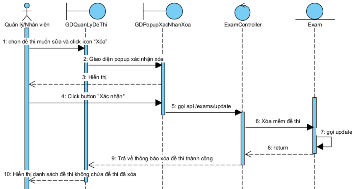
Hình 2.72 Biểu đồ tuần tự chức năng xóa đề thi
