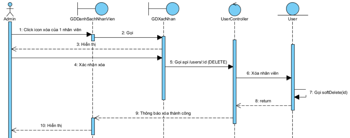
Hình 2.59 Biểu đồ tuần tự chức năng xóa nhân viên
