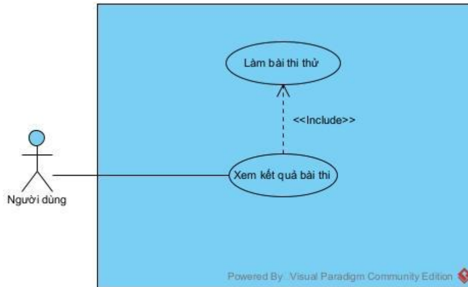
Hình 2.10 Biểu đồ use case chi tiết module xem kết quả thi
