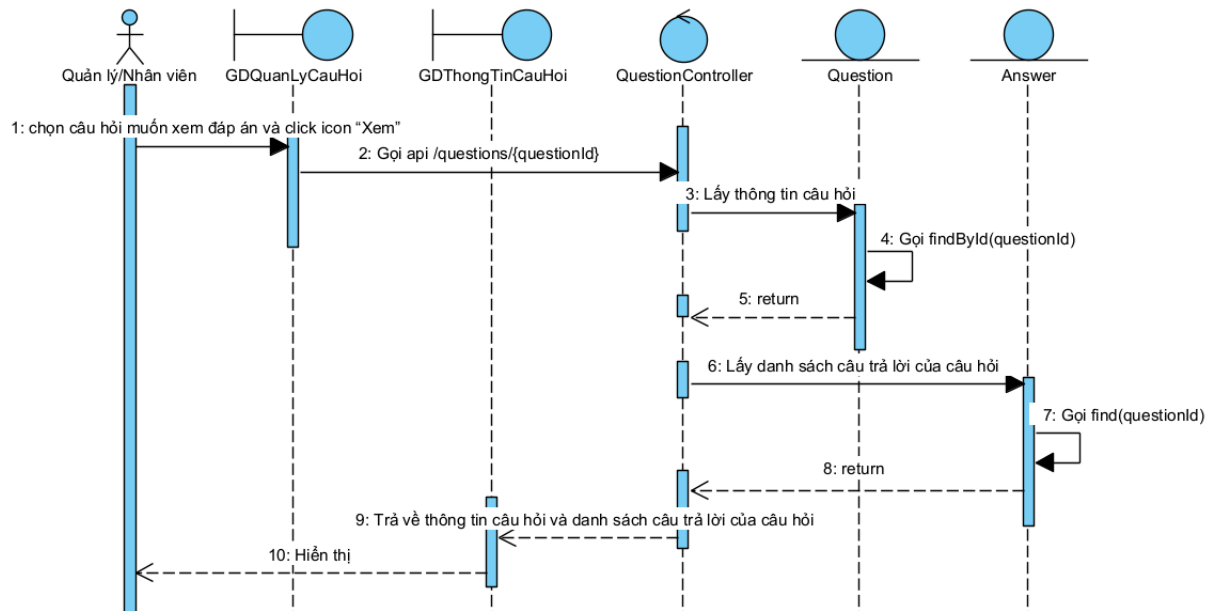
Hình 2.78 Biểu đồ tuần tự chức năng xem danh sách đáp án
