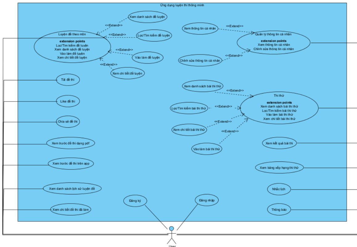
Hình 2.1 Biểu đồ use case tổng quát của ứng dụng luyện thi trực tuyến
