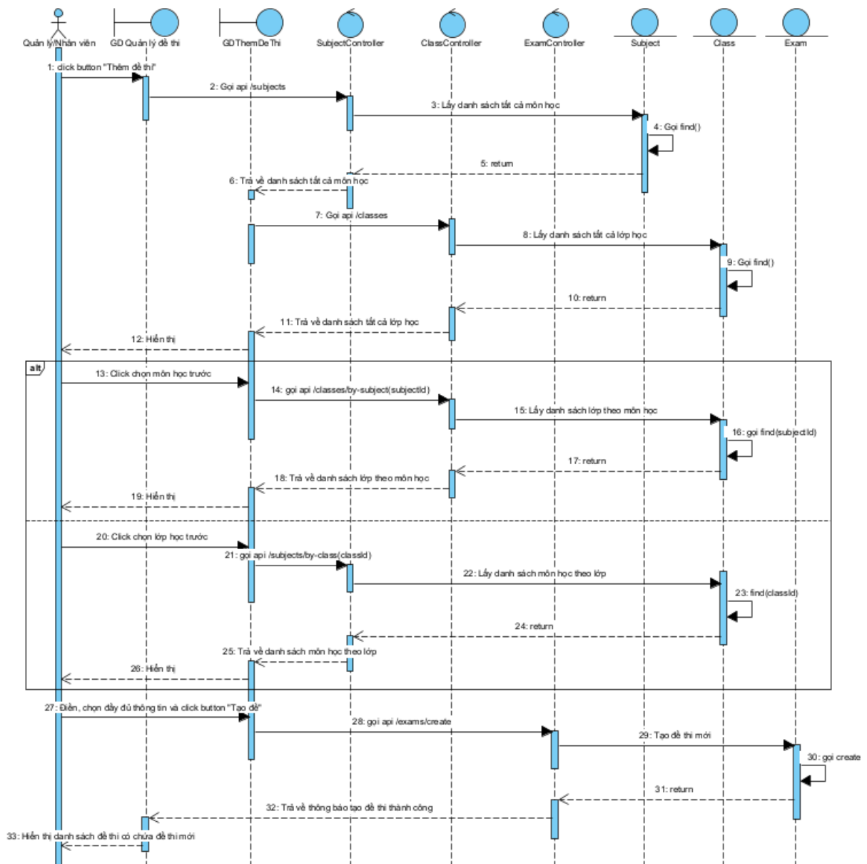
Hình 2.70 Biểu đồ tuần tự chức năng thêm đề thi
