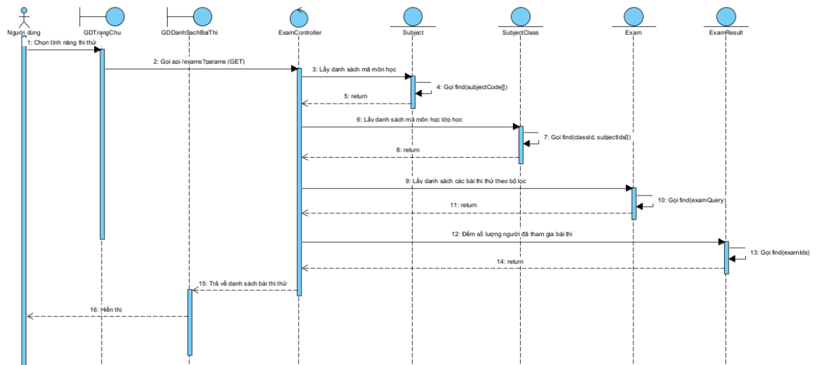
Hình 2.36 Biểu đồ tuần tự chức năng xem danh sách bài thi thử
