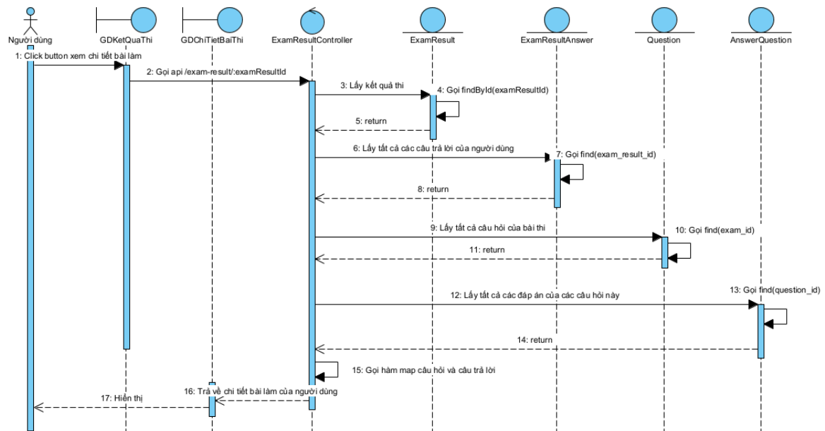
Hình 2.40 Biểu đồ tuần tự chức năng xem chi tiết bài đã làm
