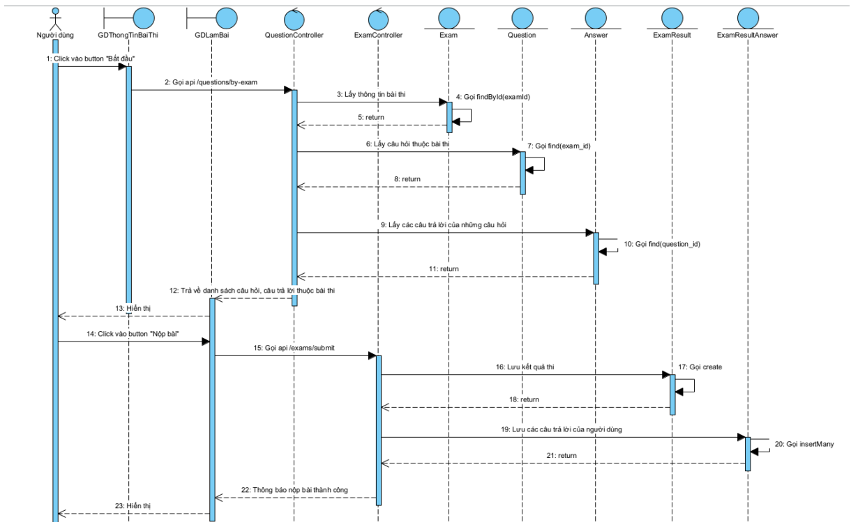
Hình 2.38 Biểu đồ tuần tự chức năng làm bài thi thử
