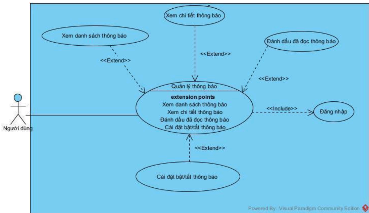
Hình 2.14 Biểu đồ use case chi tiết module quản lý thông báo
