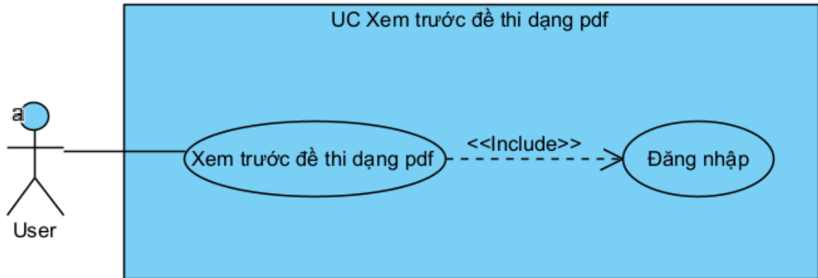
Hình 2.6 Biểu đồ use case chi tiết module xem trước đề thi dạng pdf
