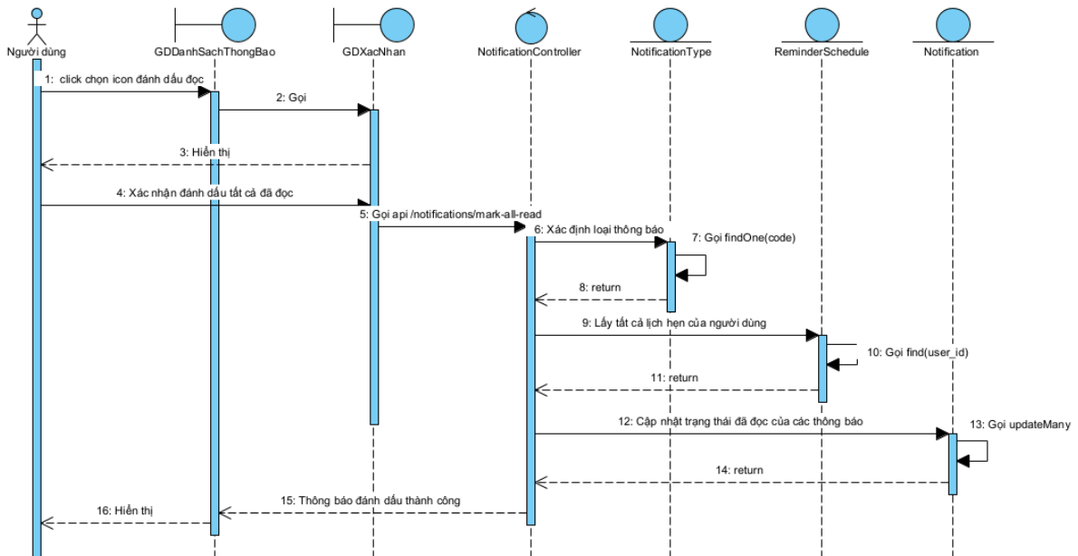
Hình 2.49 Biểu đồ tuần tự chức năng đánh dấu tất cả thông báo đã đọc
