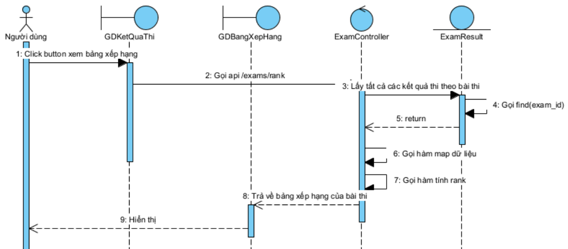
Hình 2.41 Biểu đồ tuần tự chức năng xem bảng xếp hạng
