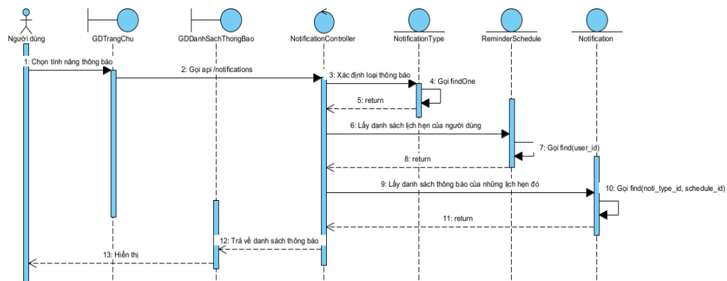
Hình 2.47 Biểu đồ tuần tự chức năng xem danh sách thông báo
