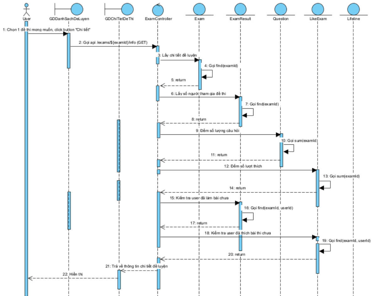
Hình 2.26 Biểu đồ tuần tự xem chi tiết đề luyện
