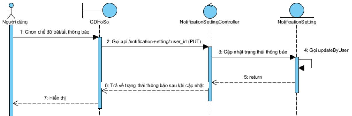
Hình 2.50 Biểu đồ tuần tự chức năng cài đặt bật/tắt thông báo
