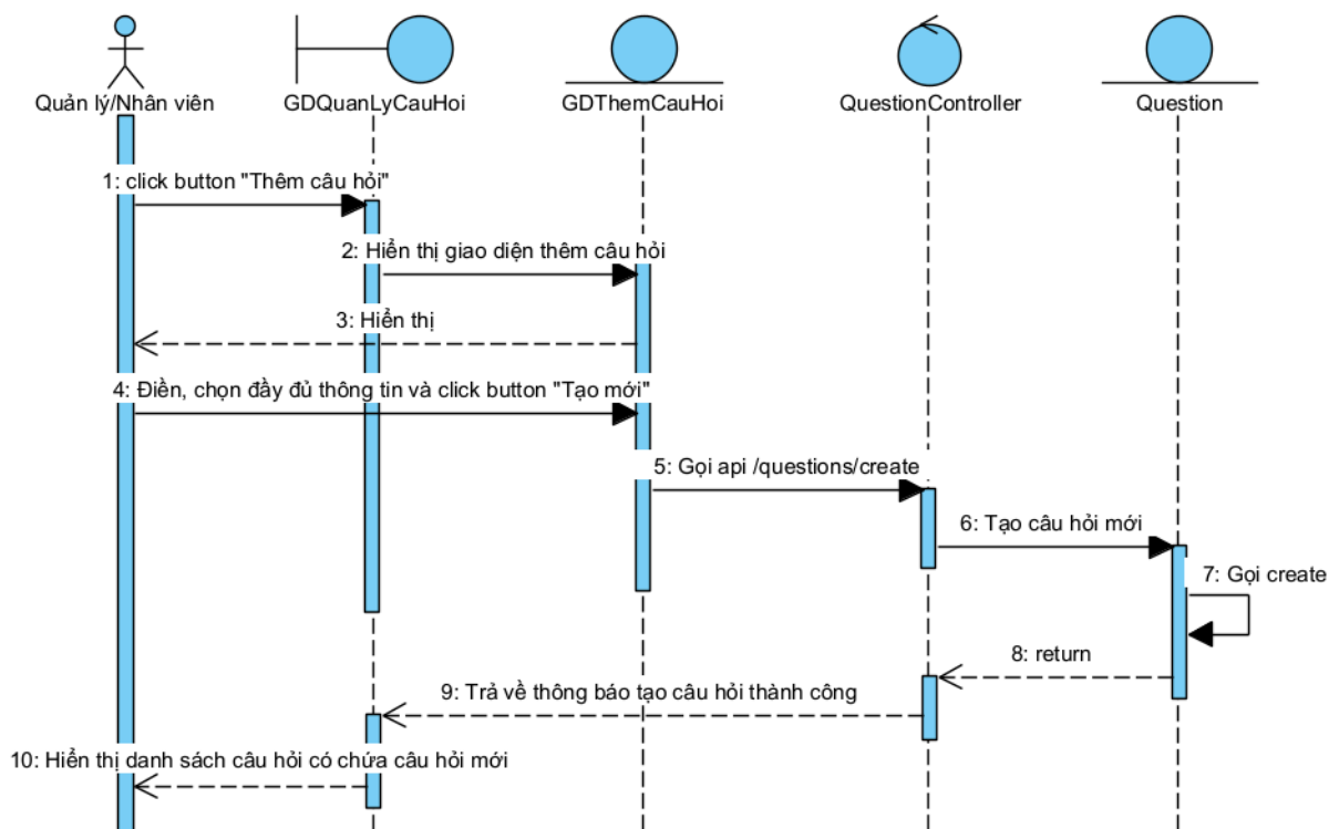
Hình 2.75 Biểu đồ tuần tự chức năng thêm câu hỏi
