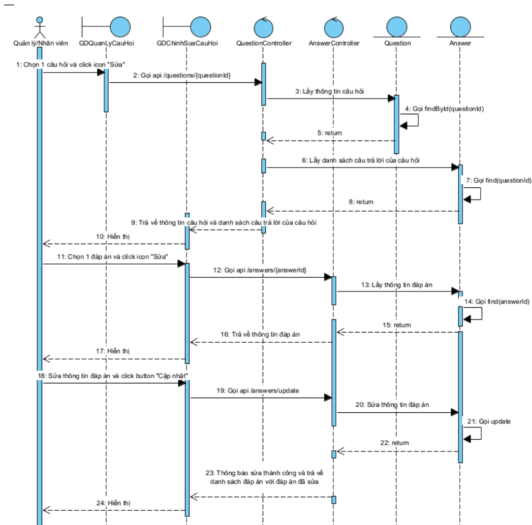
Hình 2.80 Biểu đồ tuần tự chức năng sửa đáp án
