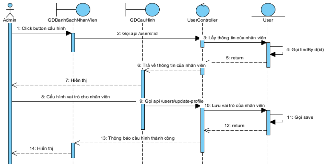
Hình 2.60 Biểu đồ tuần tự chức năng cấu hình vai trò nhân viên
