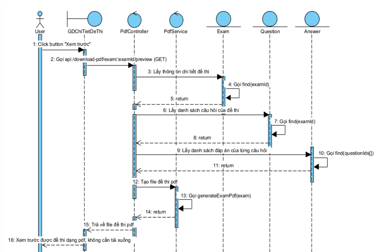
Hình 2.33 Biểu đồ tuần tự chức năng xem trước đề thi dạng pdf
