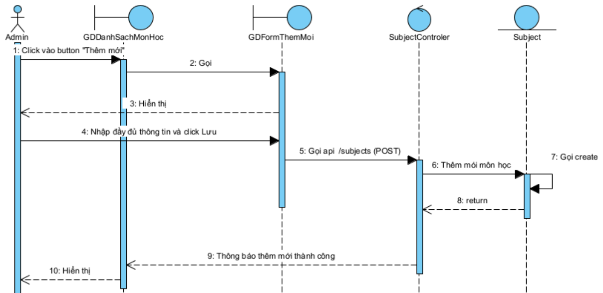
Hình 2.62 Biểu đồ tuần tự chức năng thêm môn học
