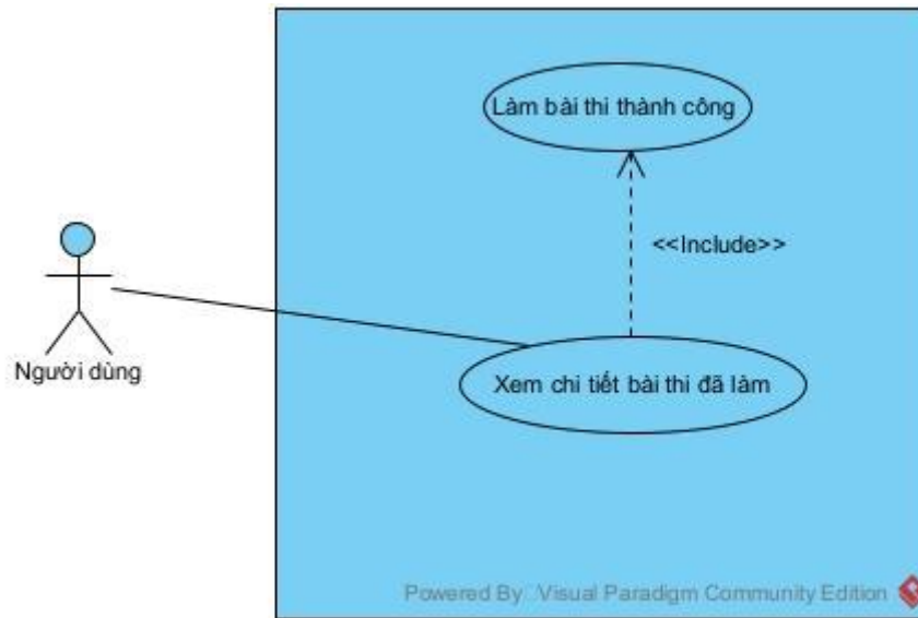
Hình 2.11 Biểu đồ use case chi tiết module xem chi tiết bài thi đã làm
