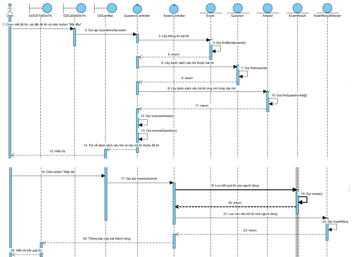
Hình 2.27 Biểu đồ tuần tự chức năng luyện đề
