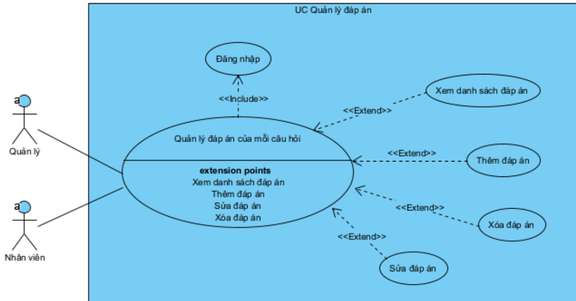
Hình 2.22 Biểu đồ use case chi tiết module quản lý câu trả lời của mỗi câu hỏi
