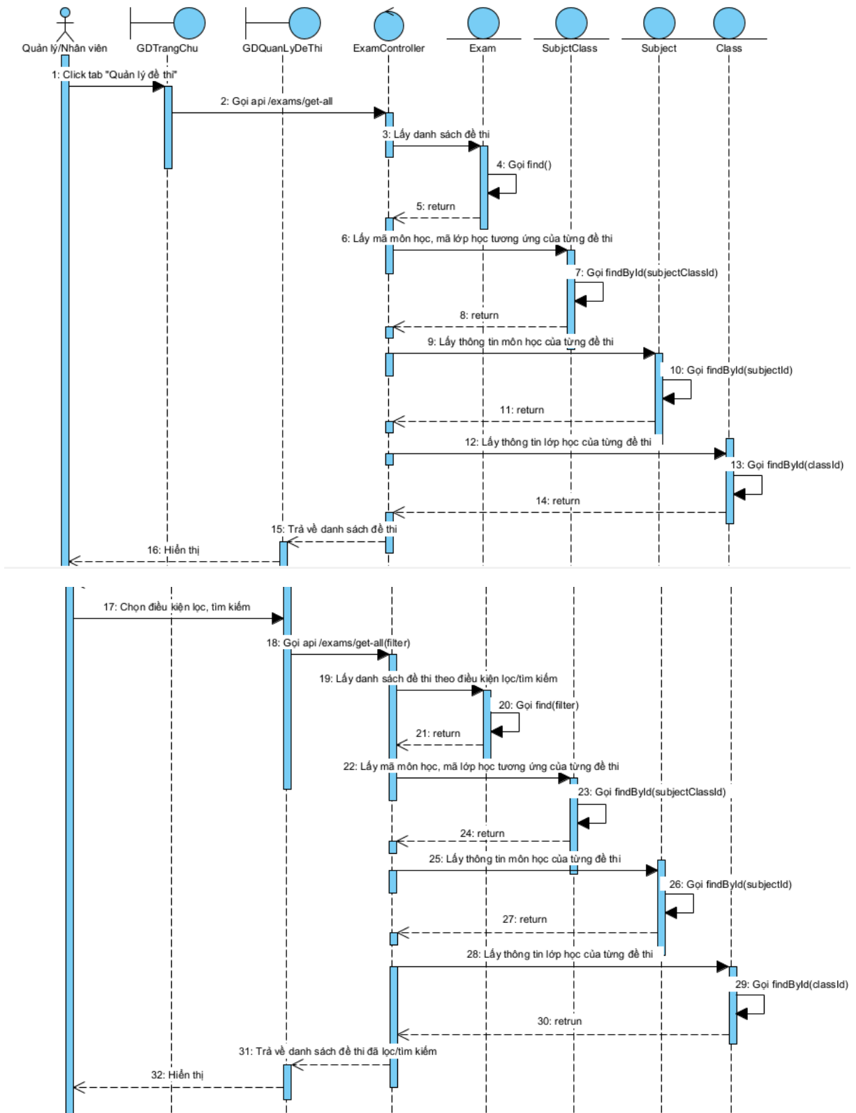
Hình 2.69 Biểu đồ tuần tự chức năng xem danh sách đề thi
