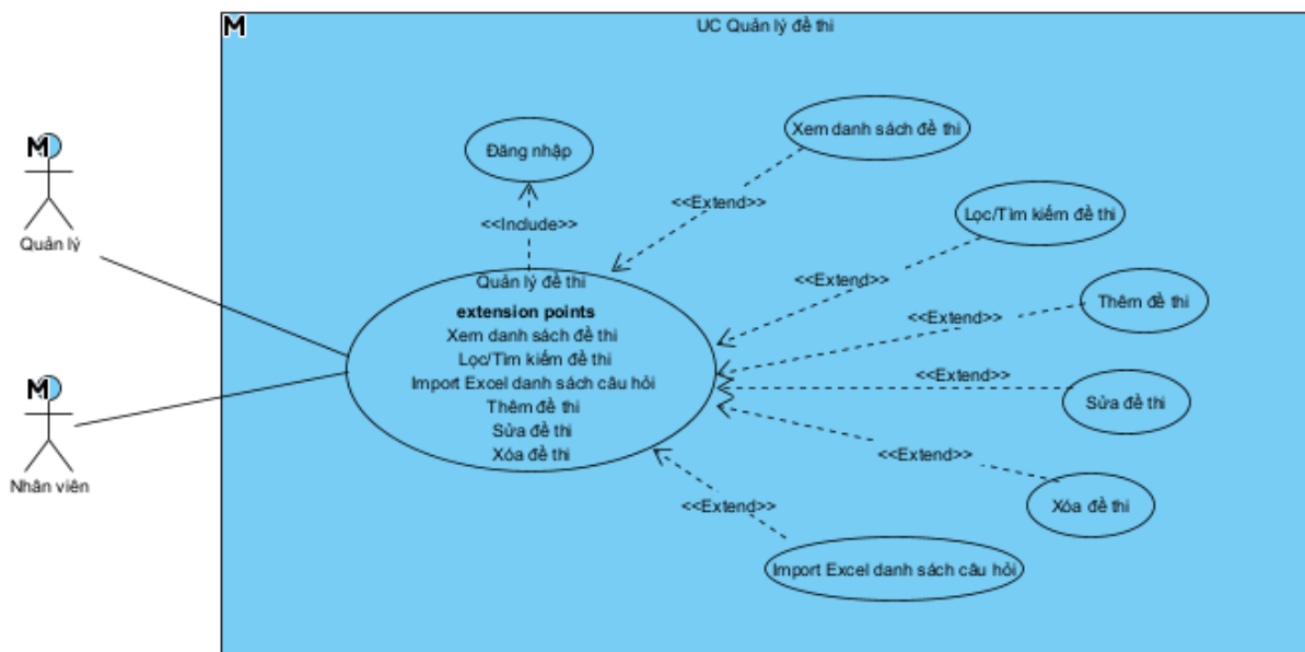
Hình 2.20 Biểu đồ use case chi tiết module quản lý đề thi
