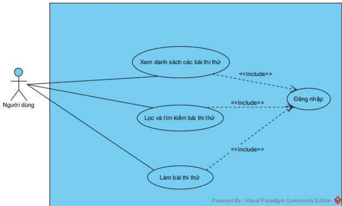
Hình 2.9 Biểu đồ use case chi tiết module thi thử
