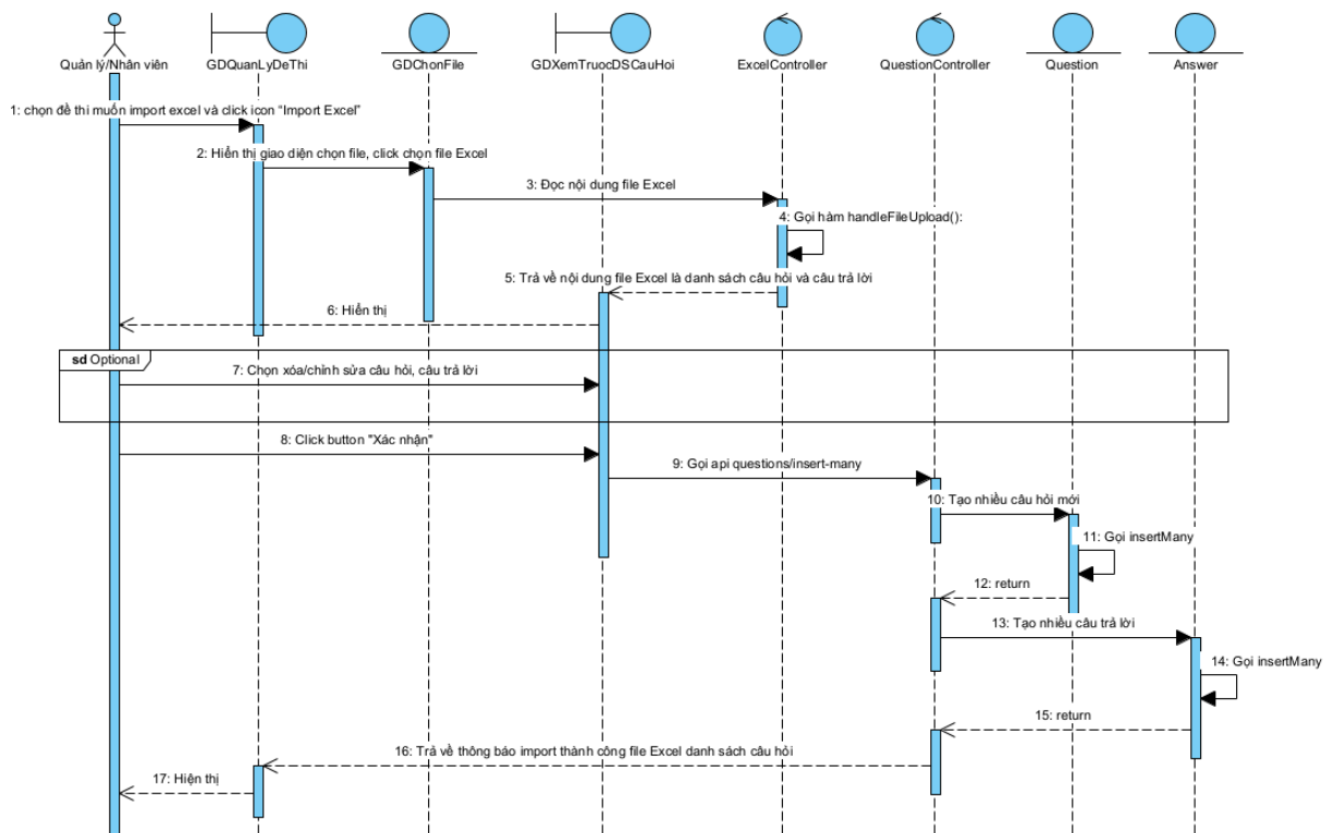
Hình 2.73 Biểu đồ tuần tự chức năng import Excel danh sách câu hỏi
