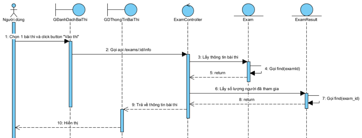
Hình 2.37 Biểu đồ tuần tự chức năng xem chi tiết bài thi thử
