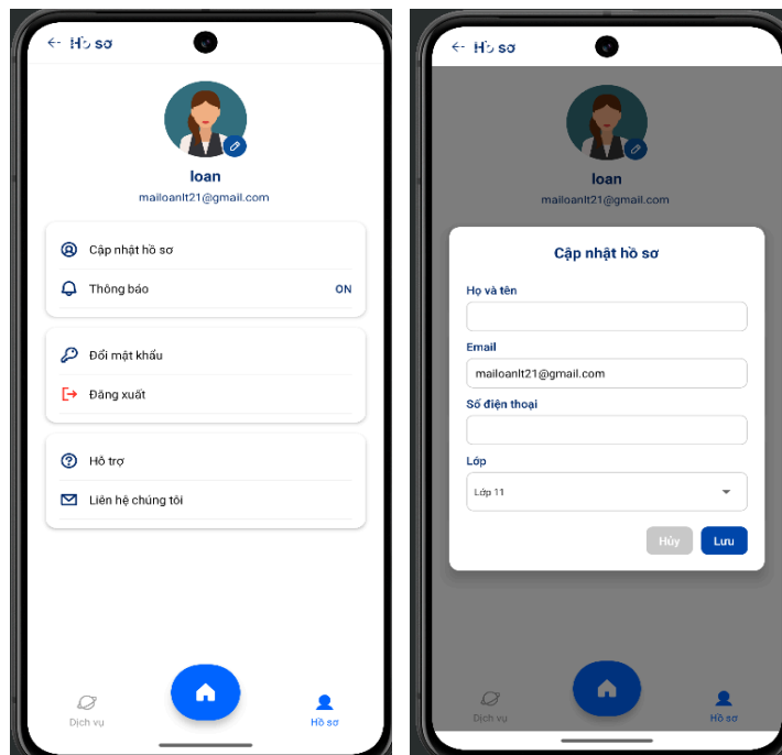
Hình 3.4 Giao diện quản lý thông tin cá nhân
