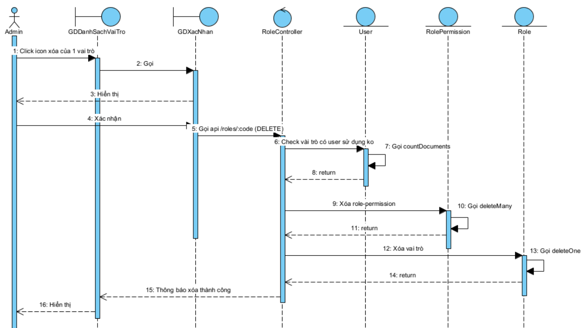
Hình 2.54 Biểu đồ tuần tự chức năng xóa vai trò
