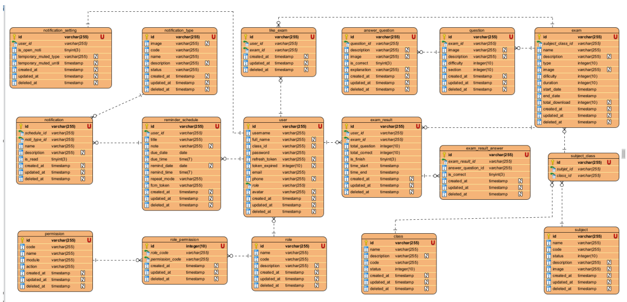
Hình 2.24 Database
