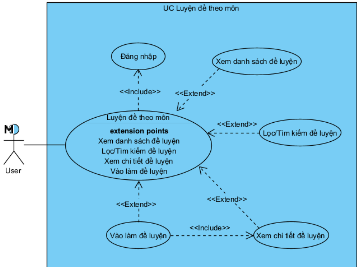
Hình 2.3 Biểu đồ use case chi tiết module luyện đề theo môn
