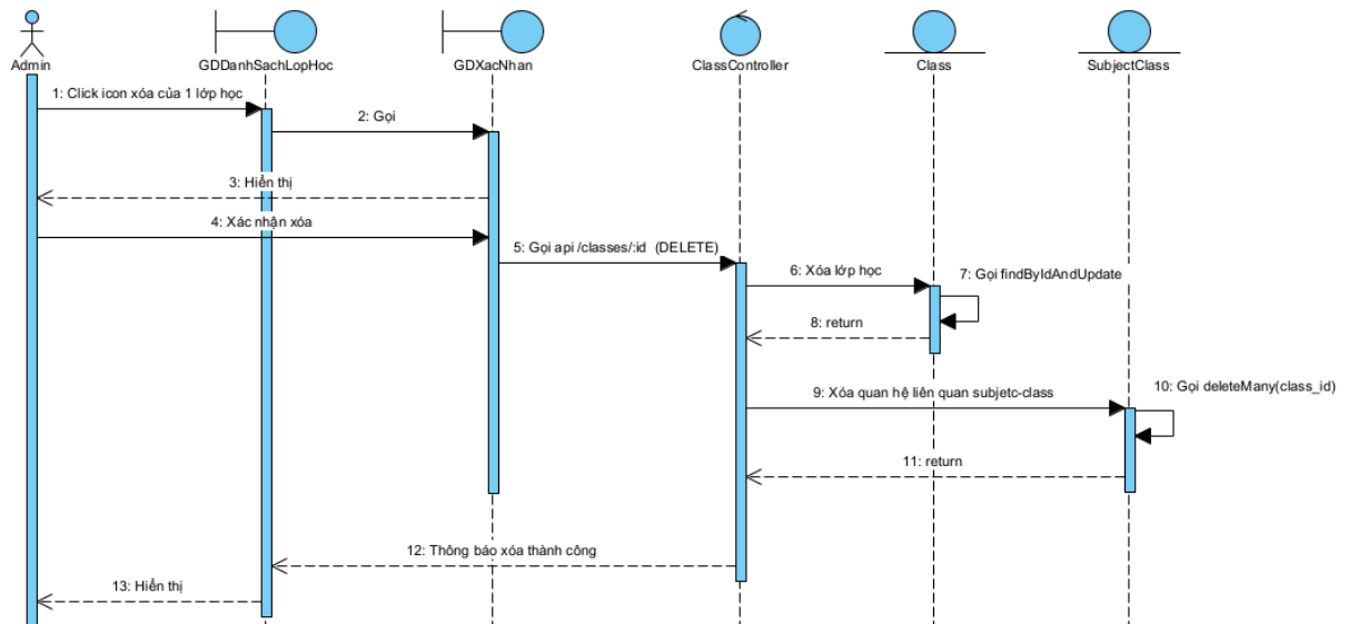
Hình 2.68 Biểu đồ tuần tự chức năng xóa lớp học
