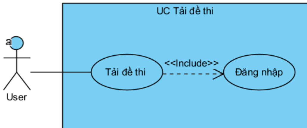
Hình 2.4 Biểu đồ use case chi tiết module tải đề thi
