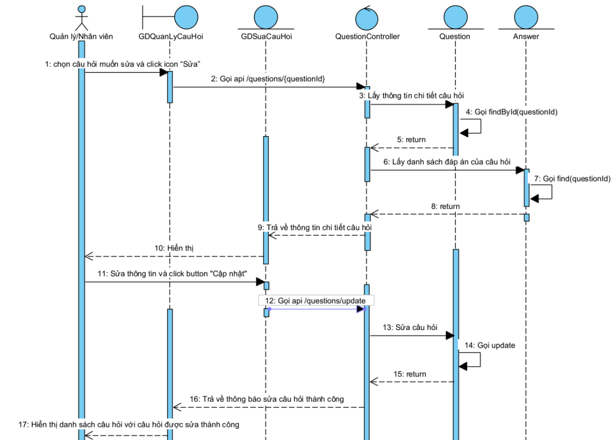
Hình 2.76 Biểu đồ tuần tự chức năng sửa câu hỏi
